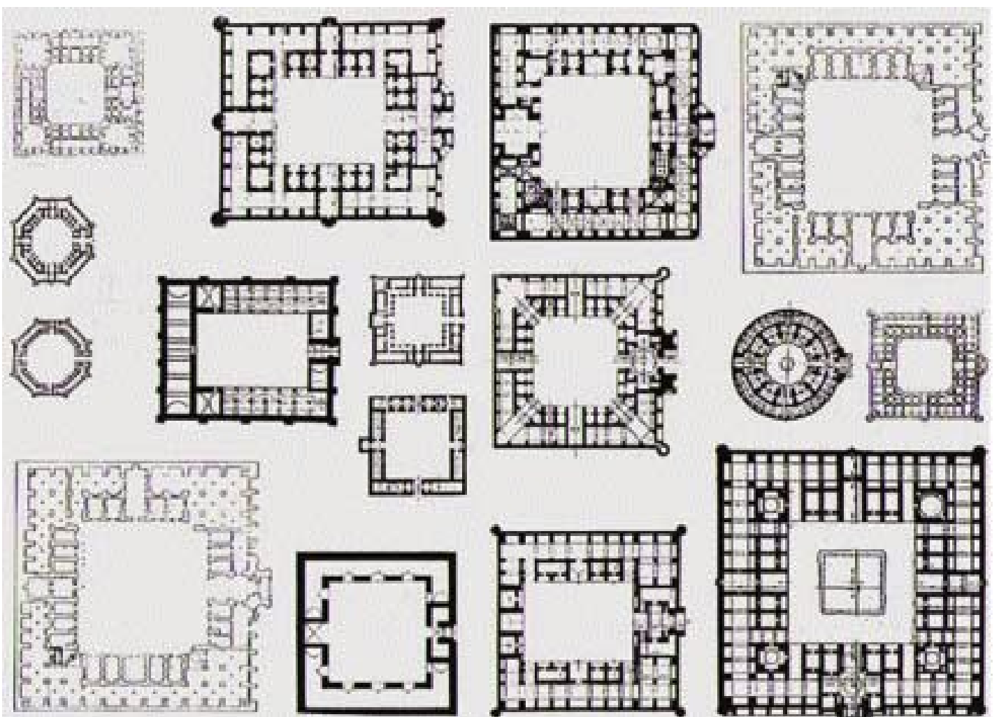
Plans comparés de divers caravansérails
